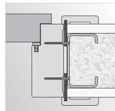
montáž na vruty do steny ze sádkokartonu
