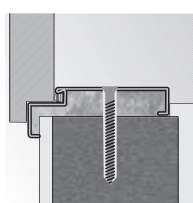
rohová záruben velká montáž pomocí šroubu
