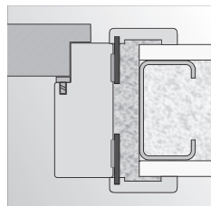
montáž na penu do steny ze sádkokartonu
