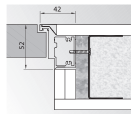
Reverzní polodrážka (otevírané dovnitř)
