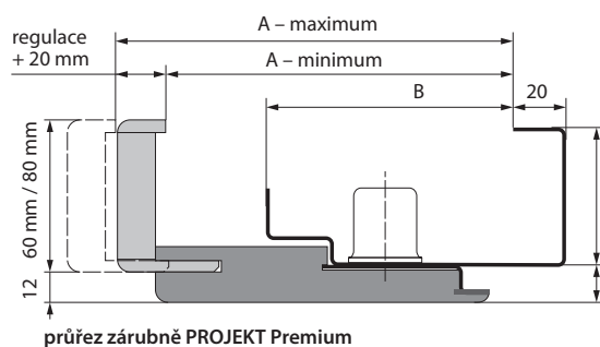
průřez zárubně PROJEKT Premium
