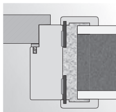
montáž na penu do zdené steny
