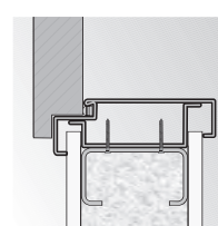
rohová záruben velká montáž na sádkokartonovou stenu
