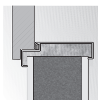
montáž bez dodatečných kotvicích prvků
