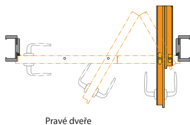
ZPŮSOB OTEVÍRÁNÍ DVEŘÍ* (pohled shora)
