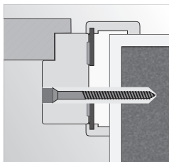
montáž na penu a kotvy do zdené steny
