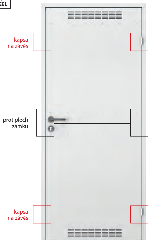
přední strana křídla
