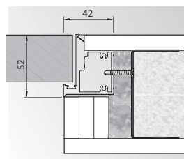
Bezpolodrážkové standard (otevírané ven)
