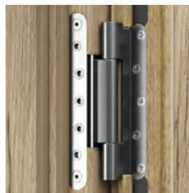
objektové závěsy
